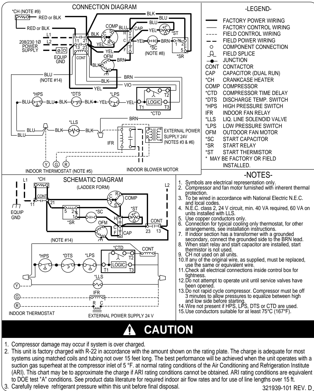
Fig. 2—38CK(C, G, S, W)060 208-230v, 1 Phase, 60 Hertz
