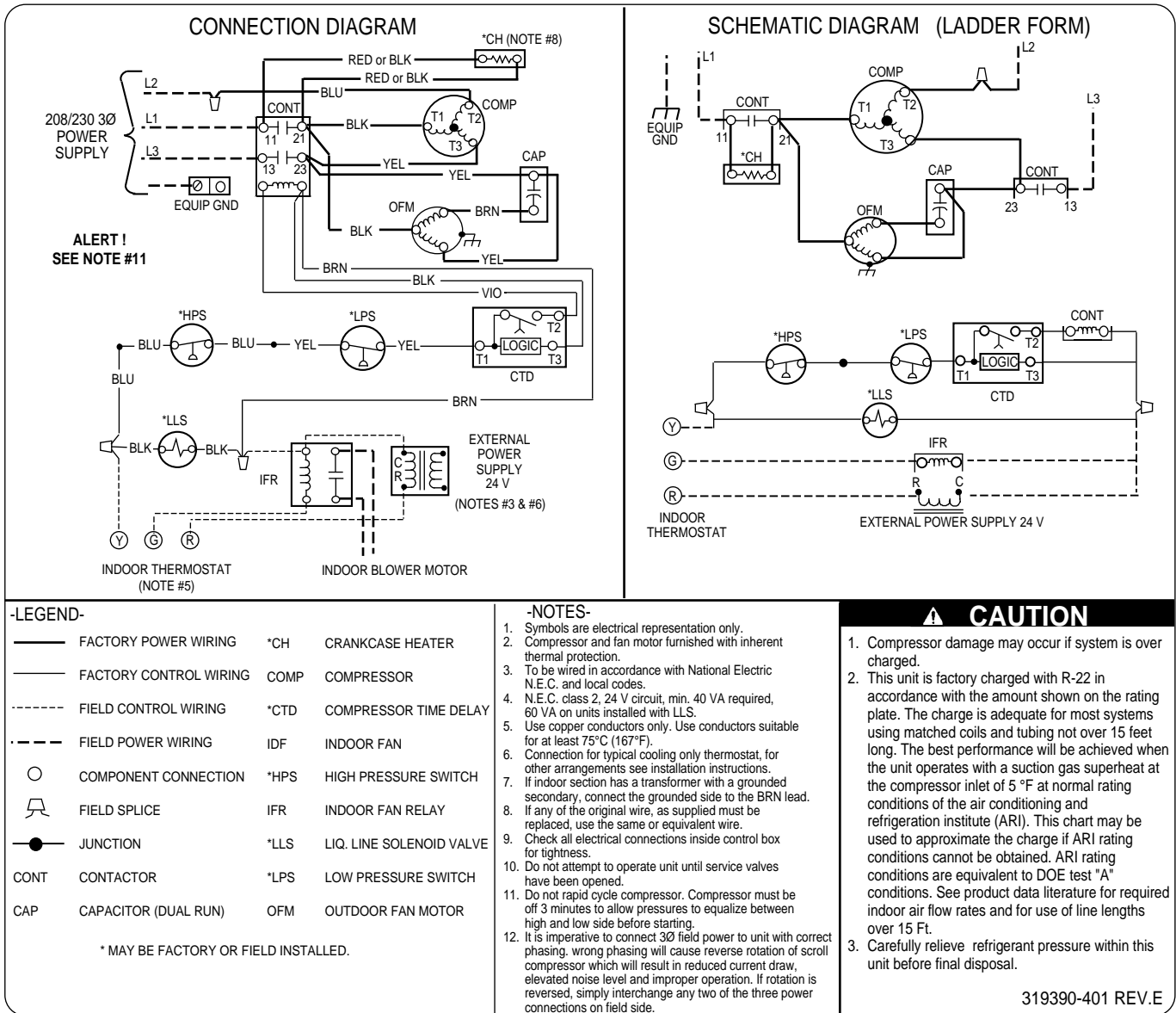
Fig. 3—38CK(C, W)030, 036, 042, 048, 060 208/230v and 38CKC036, 042, 048, 060 460v, 3 Phase, 60 Hertz
