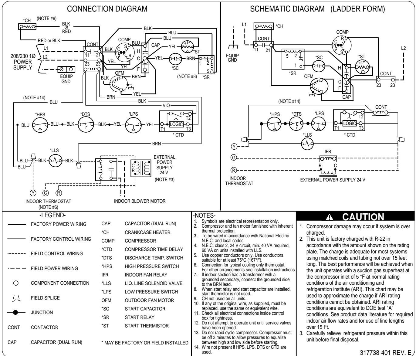
Fig. 1—38CK(C, G, S, W)018, 024, 030, 036, 042, 048 208-230v, 1 Phase, 60 Hertz
