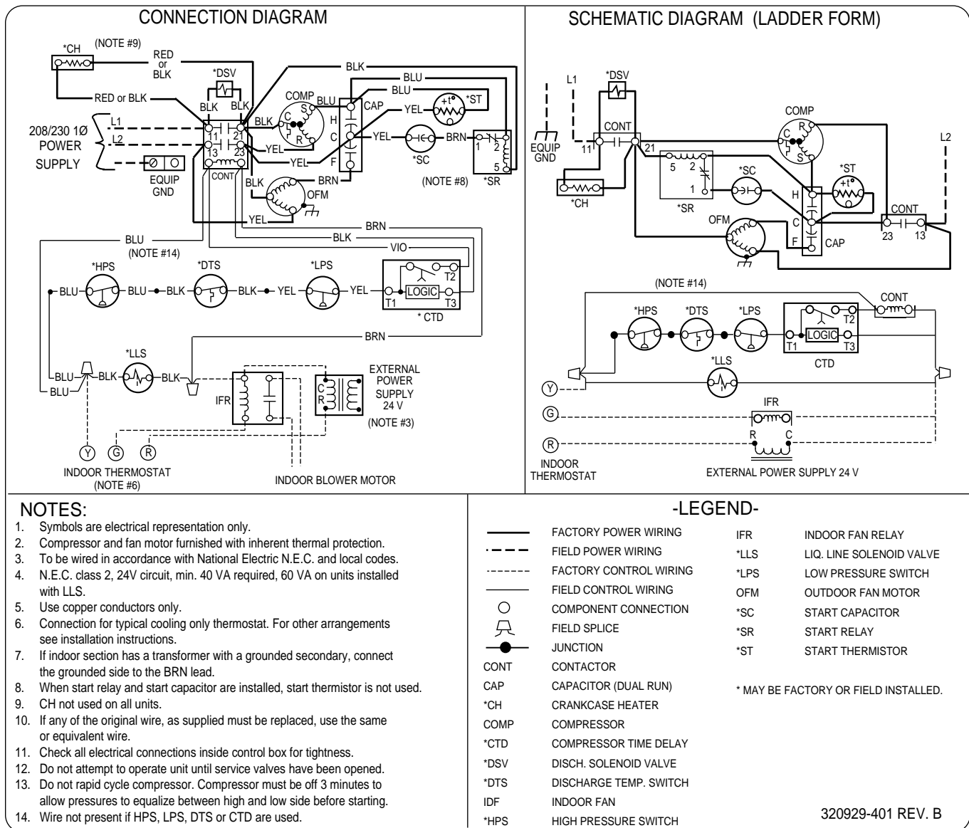
Fig. 2—38TUA060 208/230v, 1 Phase, 60 Hertz
