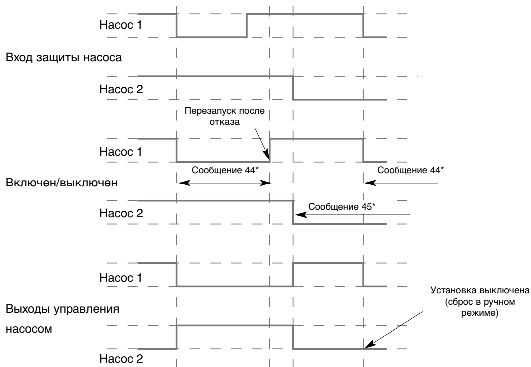
Рис. 8. Защита сдвоенного насоса
